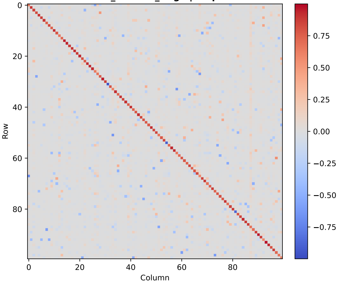
muon_random_large | step 9
